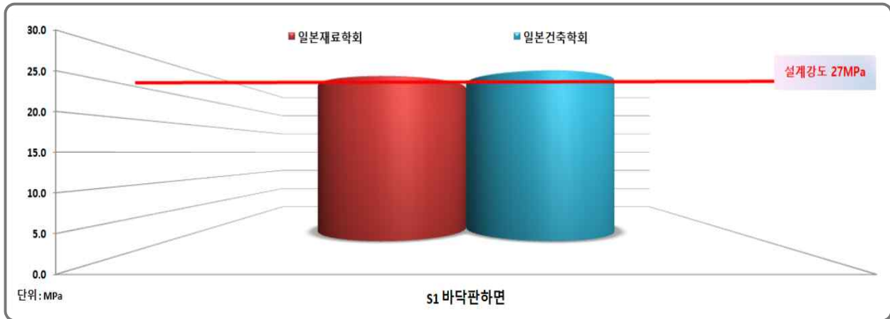
[그림 9.3.3] 반발경도법에 의한 비파괴강도 측정 결과-상부구조(바닥판하면)
