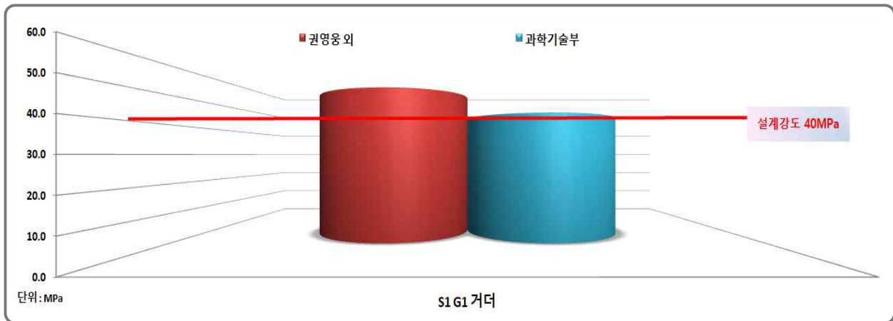
[그림 9.3.4] 반발경도법에 의한 비파괴강도 측정 결과-상부구조(거더)
