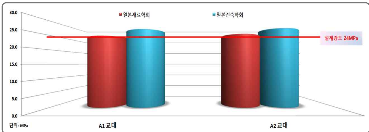
[그림 9.3.5] 반발경도법에 의한 비파괴강도 측정 결과-하부구조
