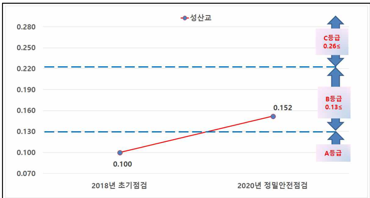
[그림 9.4.1] 성산교 상태평가 결과 비교 그래프
