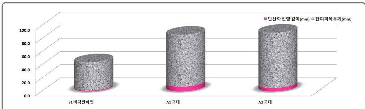
[그림 9.3.6] 탄산화깊이 및 잔여피복두께 측정결과
